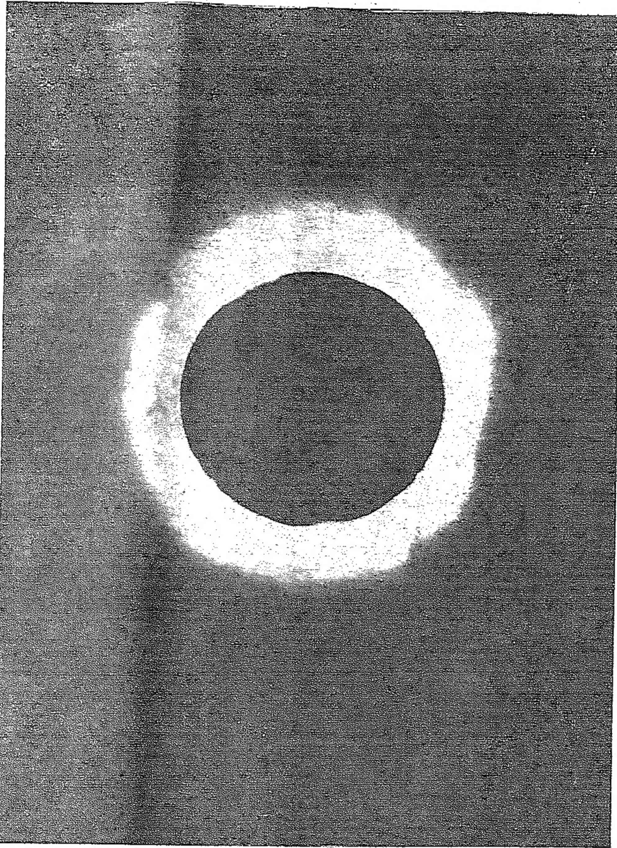
أخذت صورة لهذا الكسوف الكلي للشمس الساعية الثانية من بعد الظهر (توقيت موسكو) في قرية بورغاميش في مقاطعة الكورغان السوفياتية في الثاني والعشرين من الشهر الماضي. وقد استمر الكسوف ٢٥ ثانية، وشهده ستة من العلماء السوفييت، وثمانية من الجانب « صورة لليونانديرس »
